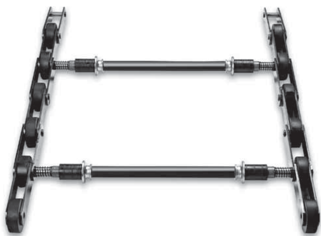
지하철 및 옥외용 엑슬형 스텝체인
